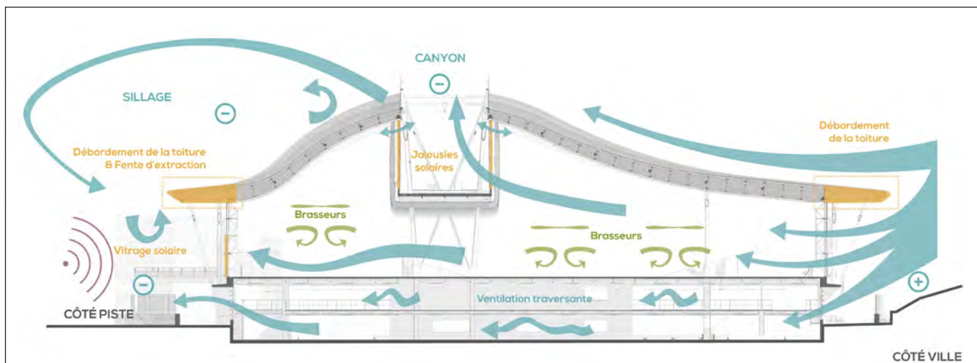
Coupe transversale extension - Sud
