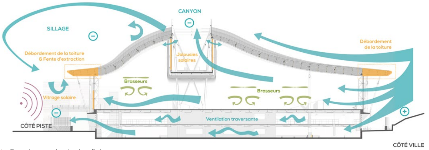
▲ Coupe transversale extension - Sud
